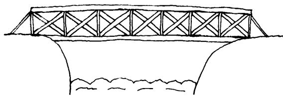
obr. 6: Most zavětrováný ondřejskými kříži
